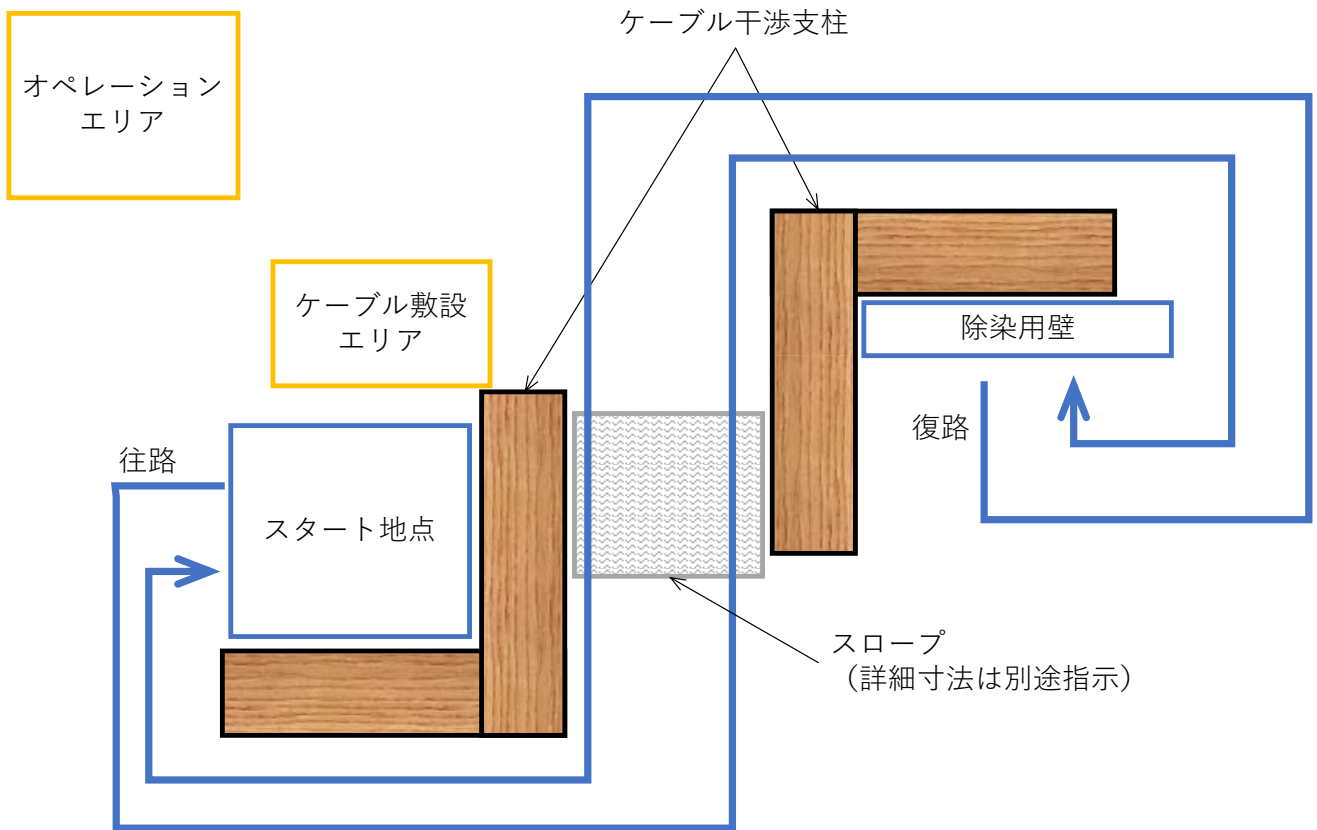
(1) 全体レイアウト及びロボットの移動経路
